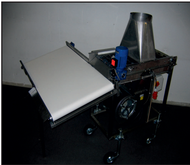
Reinigungseinheit mit "neigbarem Selektierband" (tilt belt)
